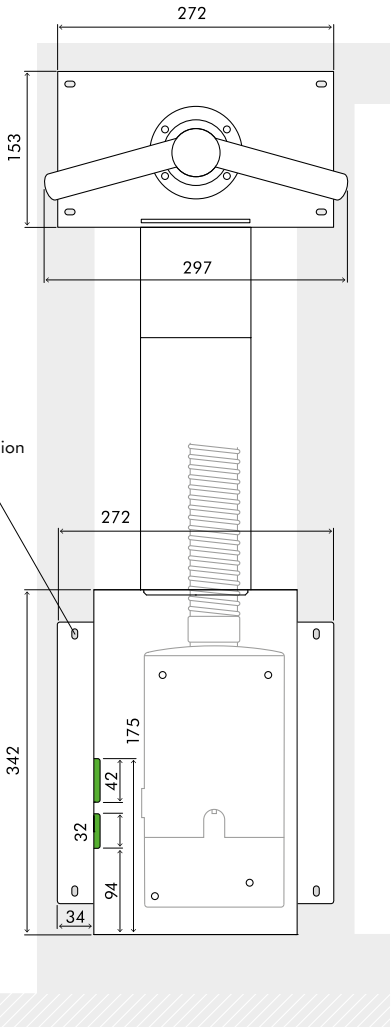
SCHEMA ARRIÈRE
