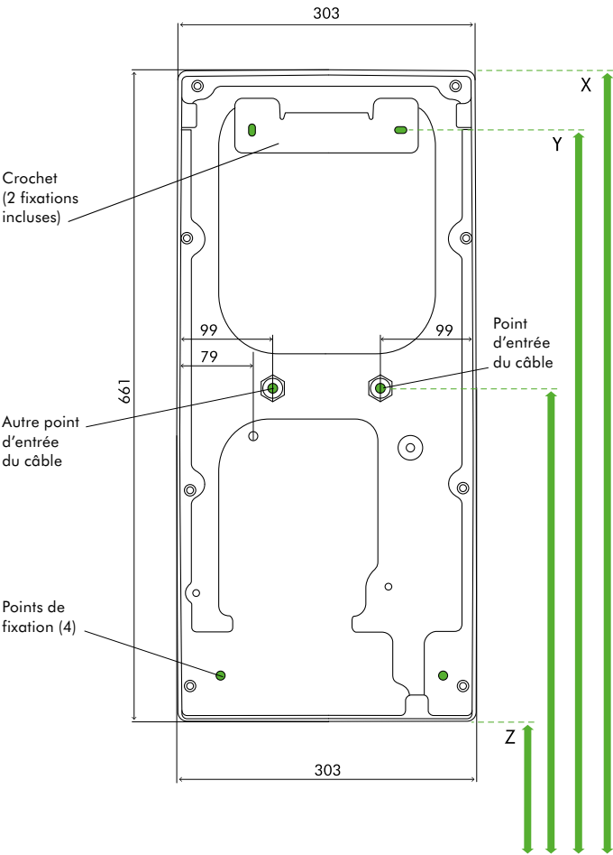
SCHEMA ARRIÈRE
