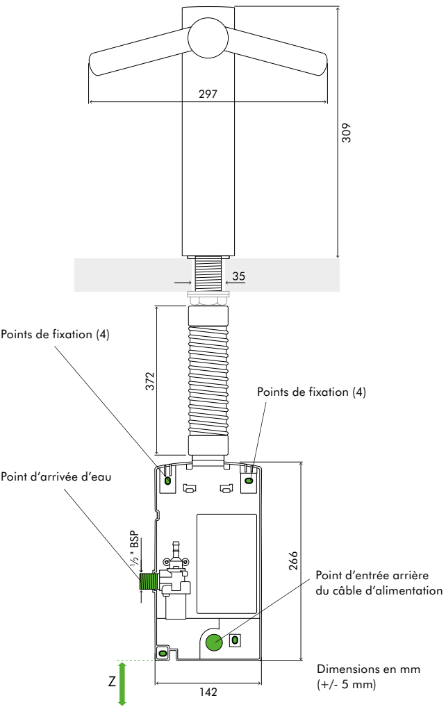
SCHEMA ARRIÈRE
