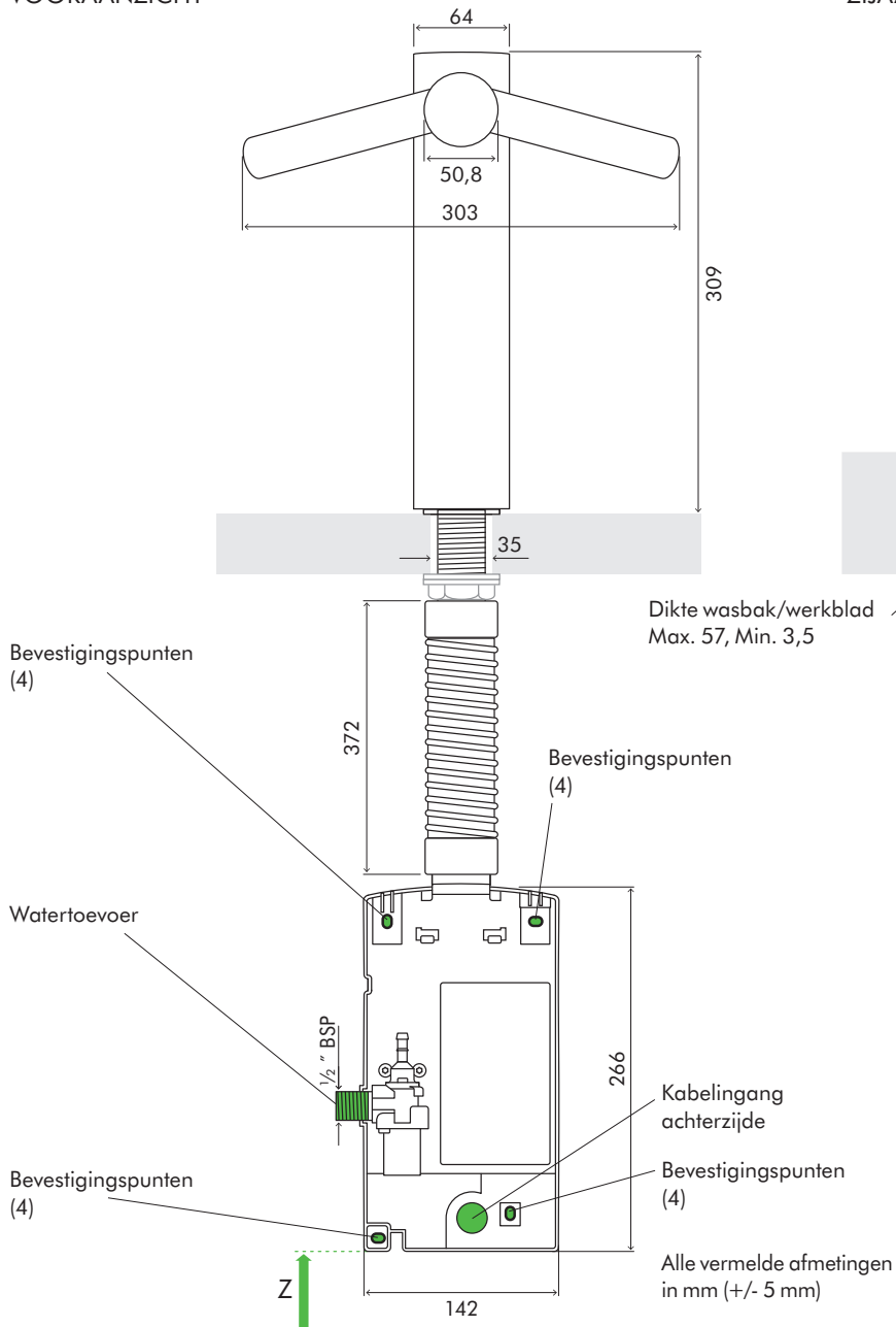
VOORAANZICHT
