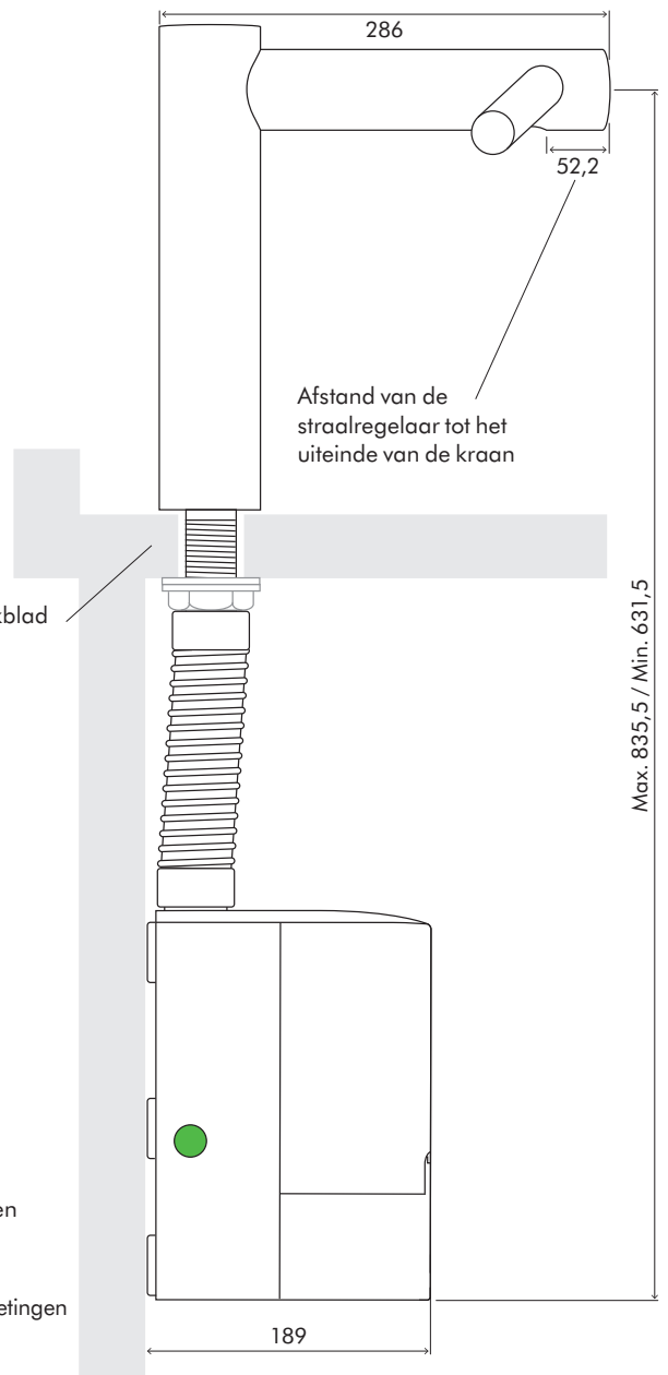
ZIJAANZICHT
